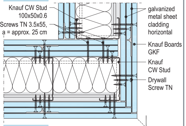
W118-D1 Corner
