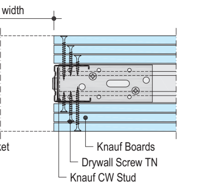
W113-E2 Door opening with Knauf CW Stud
