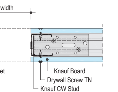
W111-E2 Door opening with Knauf CW Stud
